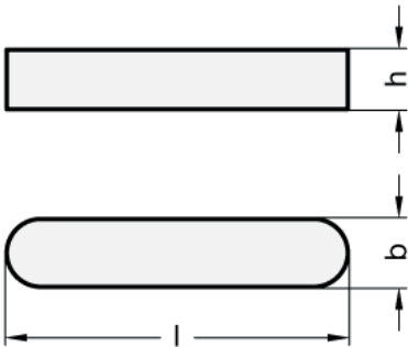
DIN 6885
